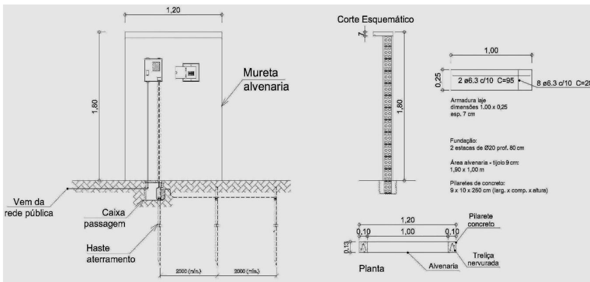
Figura 39-Projeto Mureta.
