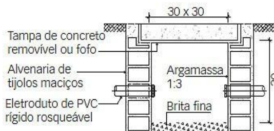
Figura 40-Caixa de passagem.
