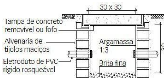
Figura 15-Caixa de passagem.
