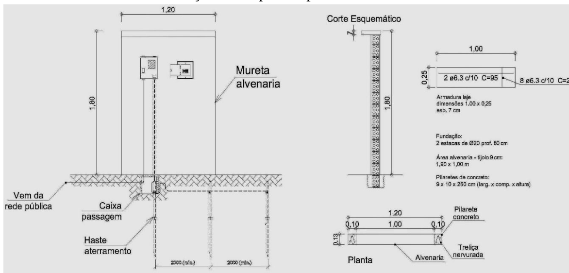
Figura 14-Projeto Mureta.
